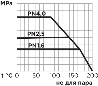
ГРАФИК ЗАВИСИМОСТИ ДАВЛЕНИЯ ОТ ТЕМПЕРАТУРЫ
